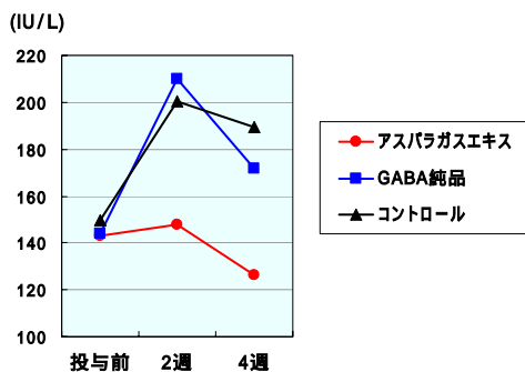
図 . GOT の変化
