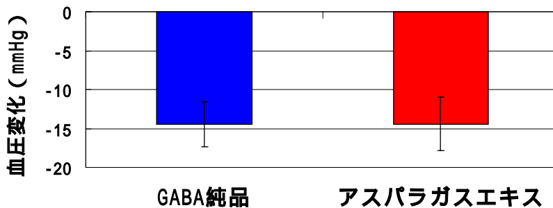
図 . 高血圧ラットを用いた血圧降下作用 (投与前と投与4時間後の比較)
