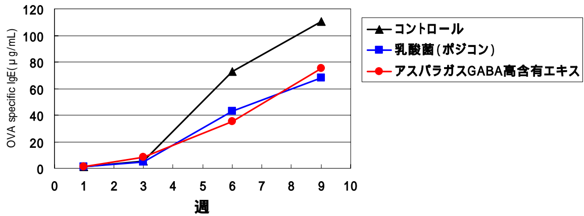
図 . 血中 OVA 特異的 IgE 濃度の経時変化 アスパラガス GABA 高含有エキスの抗アレルギー作用 (Balb/c マウス、卵白オボアルブミン (OVA) 感作)
