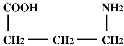
図 . GABA の構造
