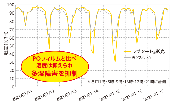
■湿度性能比較(冬季)
