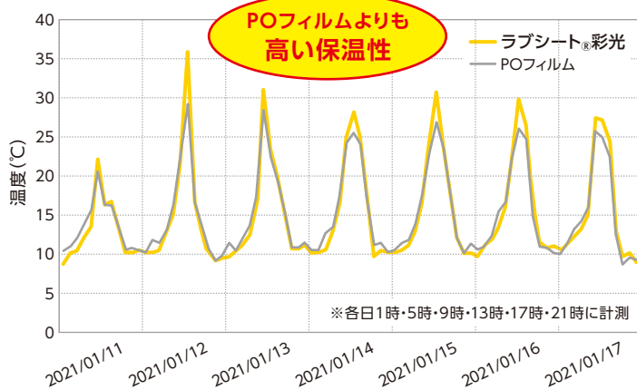
■保温性能比較(冬季)
